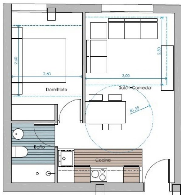
Vivienda 2,3 y 5,3 1 Dormitorio S.C: 42,32 m 2
